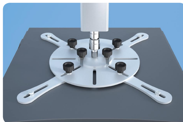
Befestigungs-Modul UNI an Beamer-Unterseite
