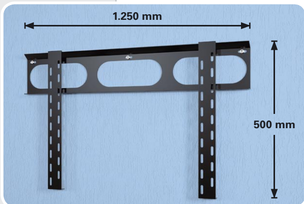
Plasma-Wandhalter ab 50"
