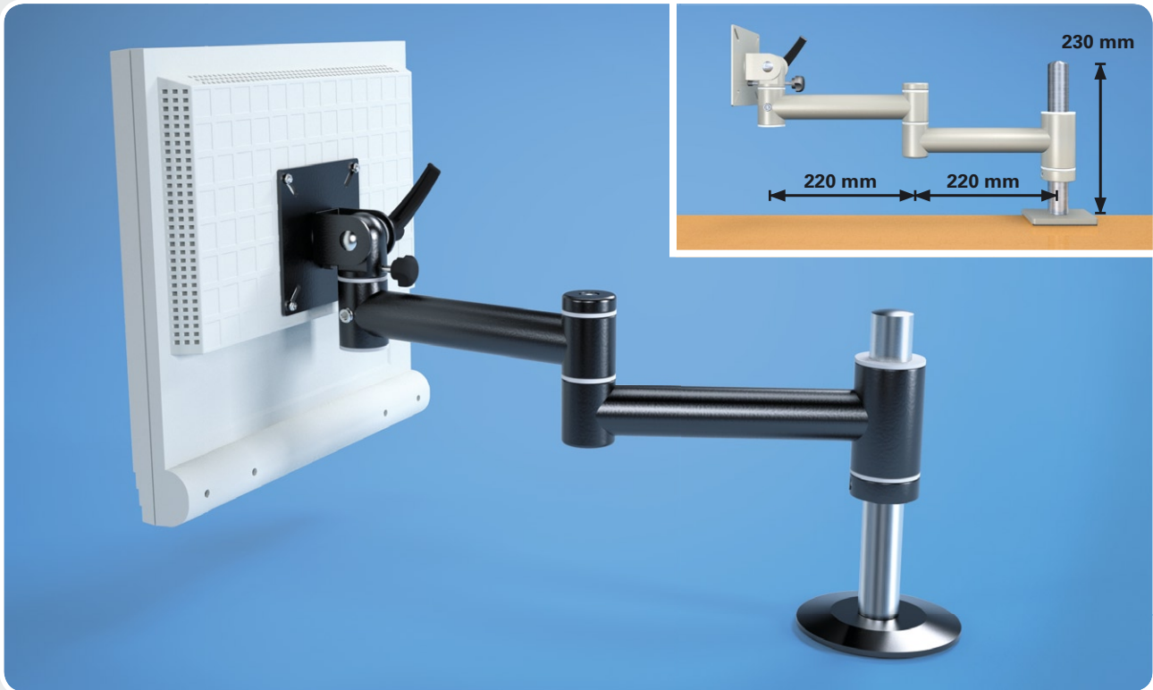
ErgoDesk® TFT-Vario mit Einbau-Adapter ohne Kabelauslass
